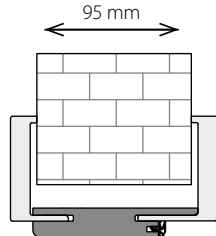
minimální rozsah regulace po zkrácení pera záklopu
