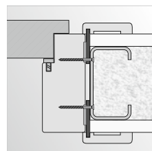
montáž pomocí šroubů do stěny SDK
