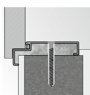
záruběň Rohová VELKÁ montáž pomocí hmoždinek
