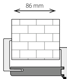
minimální rozsah regulace po zkrácení pera záklopu
