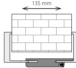
maximální rozsah regulace bez zkrácení pera záklopu
