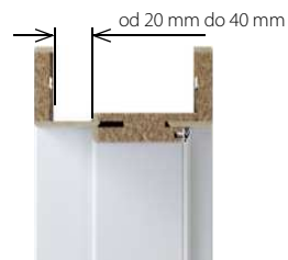
zárubeň s prodlouženým perem volitelně za příplatek
