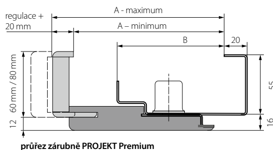
průřez zárubně PROJECT Premium
