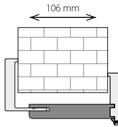
standardní rozsah regulace bez zkráceného pera záklopu
