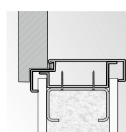
záruběň Rohová VELKÁ montáž na stěně SDK
