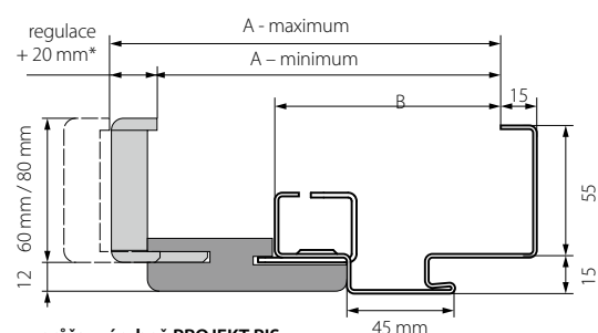
průřez zárubně PROJECT BIS
