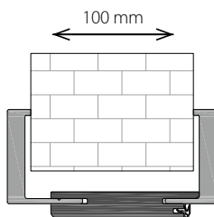
standardní rozsah regulace bez zkrácení pera záklopu
