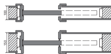
POSUVNÉ SYSTÉMY KOMPAKT URČENÉ PRO STĚNY O TLOUŠŤCE 100 A 150 MM
