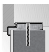
záruběň Rohová VELKÁ montáž pomocí hmož- dínek
