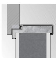
montáž bez dalších kotevnic prvků
