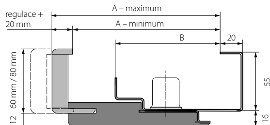
průřez zárubně PROJEKT Premium
