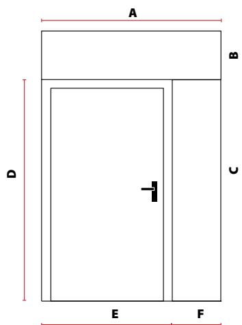
PORTA THERMO - ROZMĚROVÁ ÚPRAVA CO 10 mm
