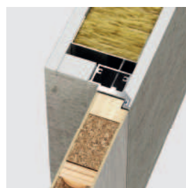
Reverzní falc (otvírání dovnitř) - levé dveře
