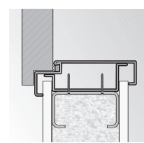
zárubeň Rohová VELKÁ montáž na stěně SDK
