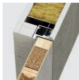
Bezfalcový standard (otvírání ven) - pravé dveře
